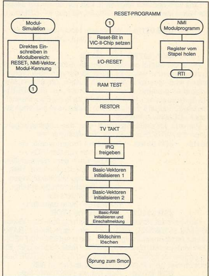
Bild 46. Das Flußdiagramm zum Listing 6, Modulsimulation
