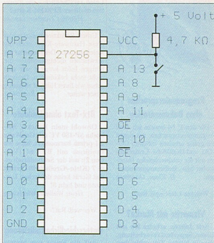
Per Schalter läßt sich im EPROM-Speicher umschalten (z.B. zwischen zwei Betriebssystemen)
