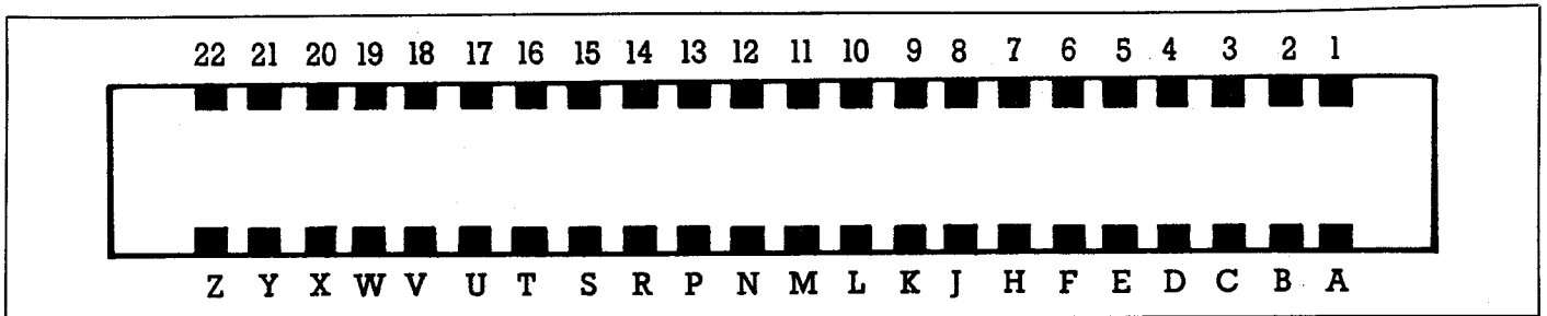
Der Expansion-Port des C 64 — von hinten gesehen
