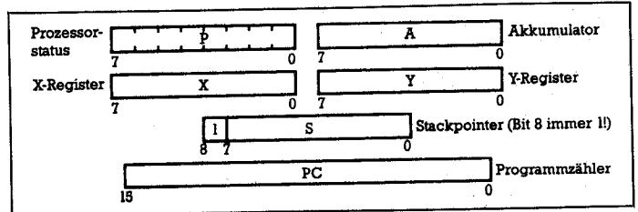
Registersatz des 6502/6510
