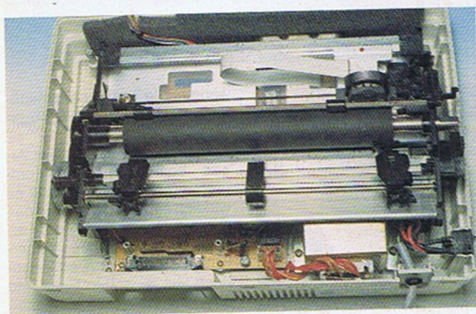
Im Inneren des Druckers wird gute Handwerksarbeit sichtbar
