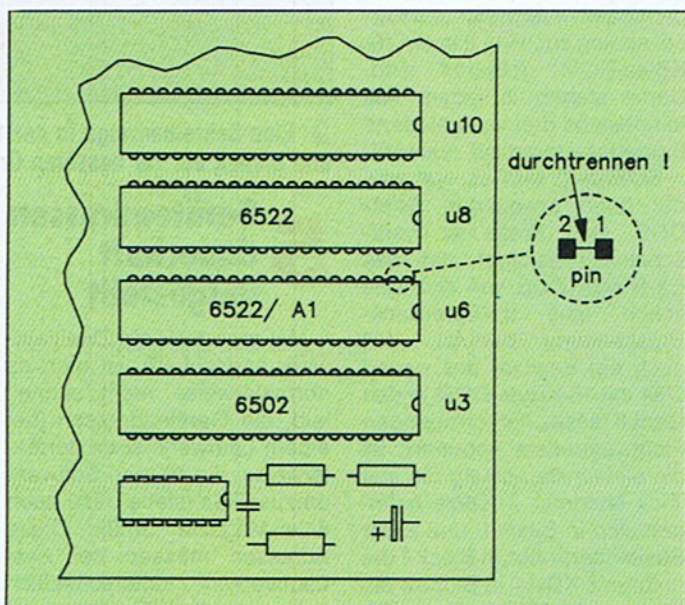
6 Der zum Anschluß eines Parallelkabels an die 1541 II relevante Ausschnitt der Elektronik. Beachten Sie, daß auf der Platinerückseite eine Leiterbahn getrennt werden muß.
