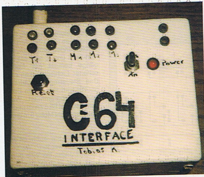
1 Das fertige Interface (hier nur provisorisch beschriftet)
