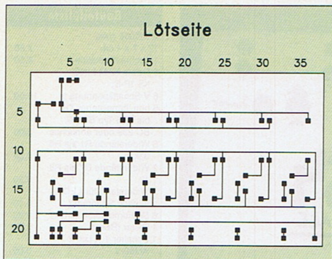
2 Lötseite der Platine, es genügt eine Lochrasterplatine
