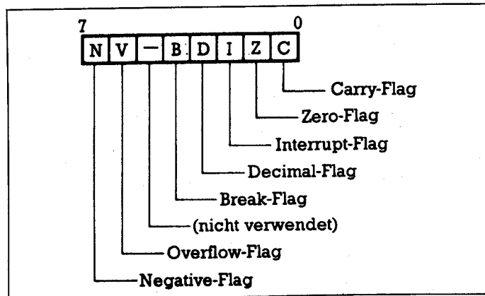
Das Flag-Register
