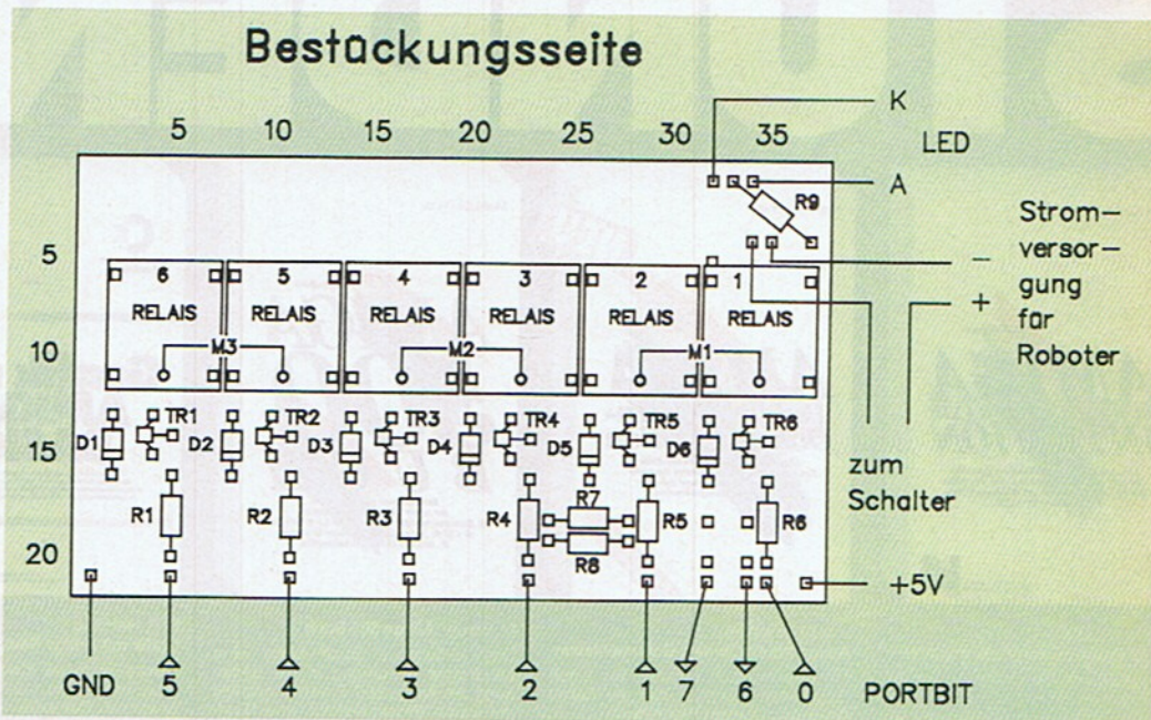
4 Bestückungsseite der Platine, man sieht, wie kompakt das ganze Gerät wird
