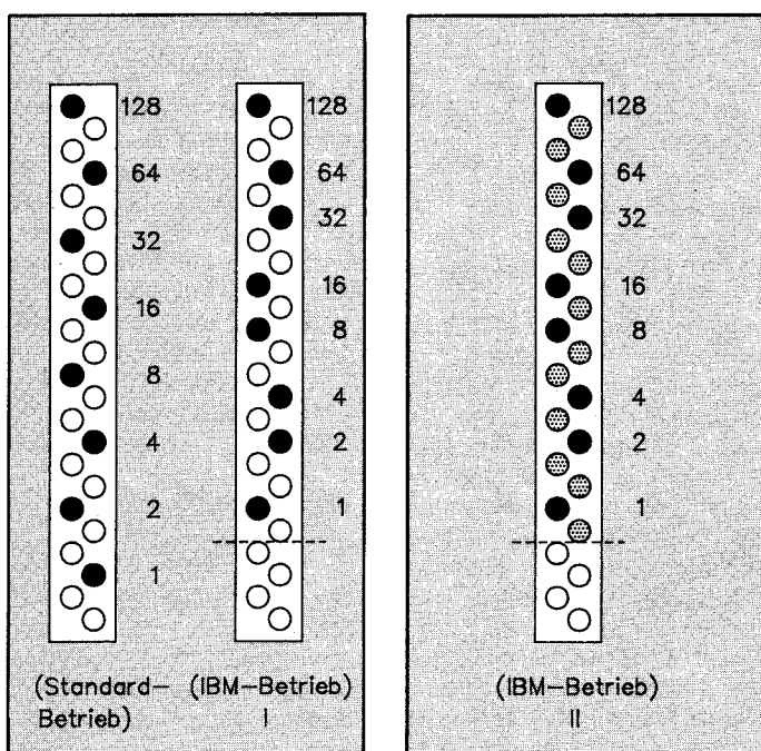
1 Die Verteilung von 8 Punkten auf 20 Nadeln
