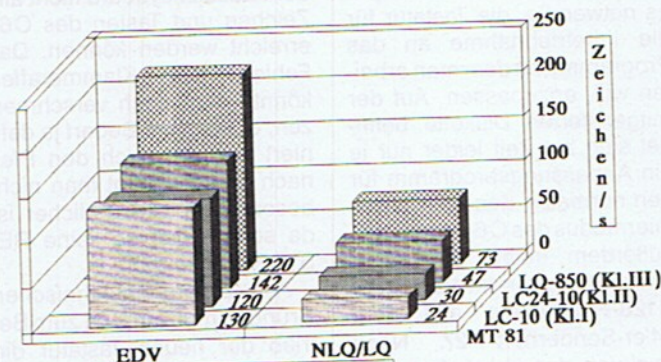
(Th. Lipp 89) Druckgeschwindigkeit
