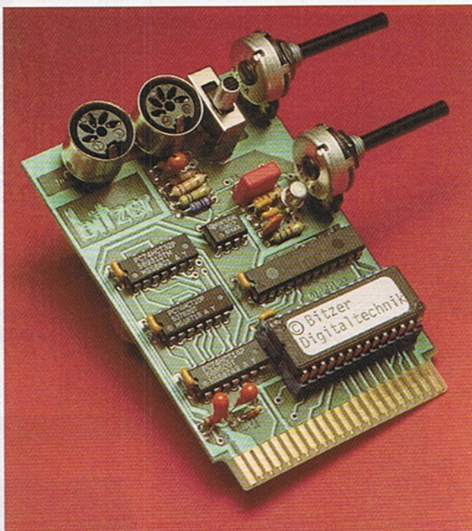
Die Digital-Analog-Platine von Bitzer Digitaltechnik
