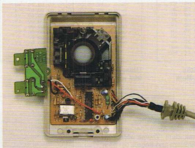
Bild 1. Das Innenleben der Commodore-Maus 1351. Deutlich zu erkennen ist der Quarz links vorne.
