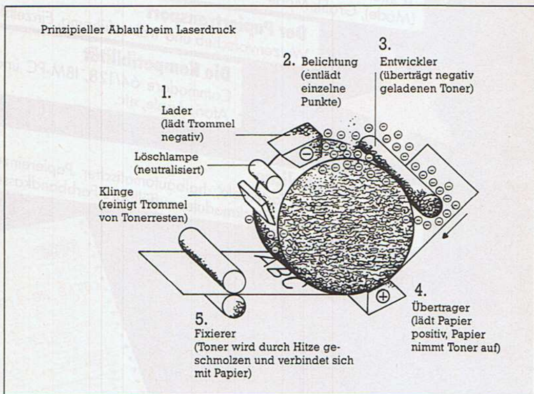
Bild 5. So arbeitet ein Laserdrucker Quelle: Sperry Technical Manual Modell 37
