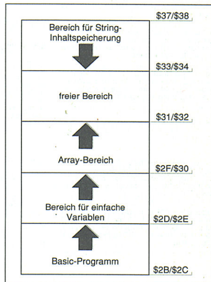
Abb. 3 Aufteilung des Basic-RAMs
