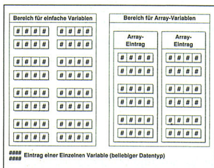
Abb. 1 Der Aufbau des Variablen-Speichers
