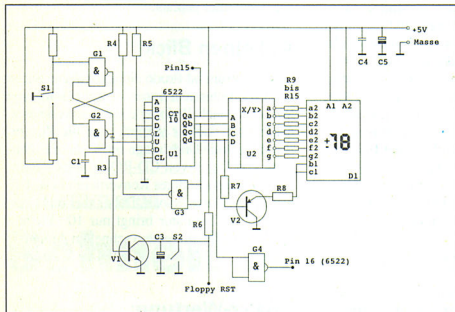
Der Anschluß an die 5-V-Leitung des Disketten-Laufwerks
