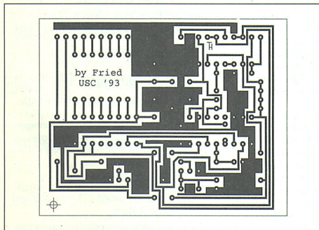
Das Platinen-Layout (links) und der Bestückungsplan - das Layout liegt als Postscript in der PCgo!-Mailbox (s. Kasten „Layout-Service“)
