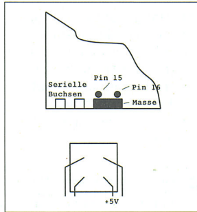
Der Anschluß an die 5-V-Leitung des Disketten-Laufwerks
