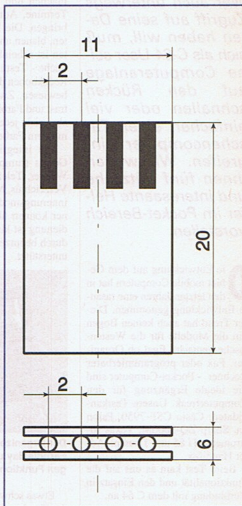
3 Der Anschlußstecker für den HP-Pocket-Computer wird mit einigen Tricks einfach nachgebaut (Maßangaben in mm)
