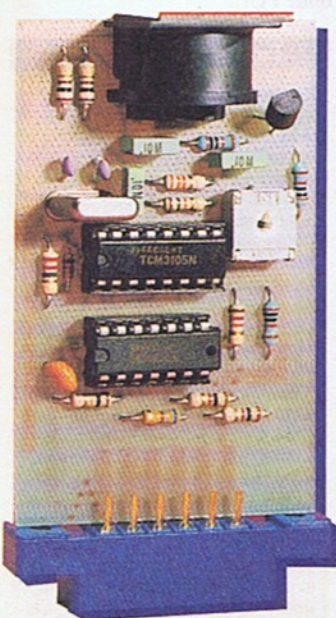
Das Spezialmodem (Lührmann-Elektronik) überträgt zwischen C 64 und dem CB-Funkgerät
