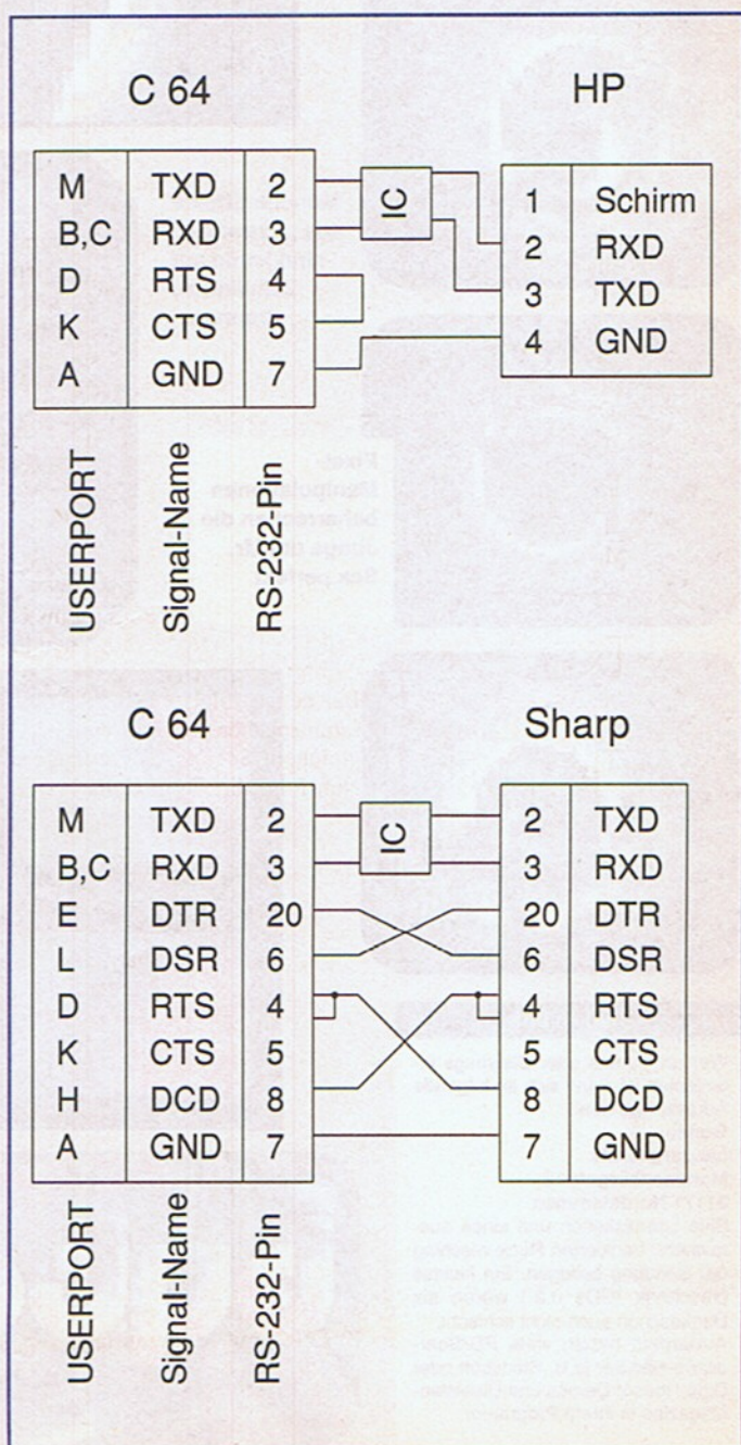
1 Die Schnittstellen der beiden Taschencomputer (oben) und die Beschaltung der Verbindungskabel (rechts)
