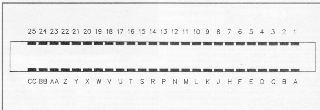
Pin-Belegung des Expansion-Port C 16/Plus/4. So präsentiert er sich dem Anwender an der Gehäuserückseite.
