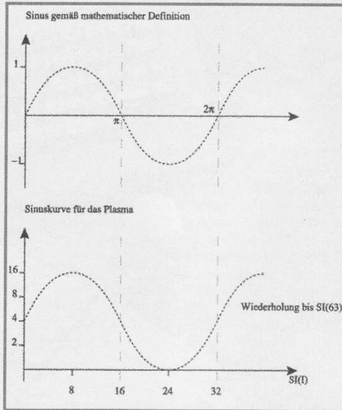
Der Vergleich zwischen herkömmlicher mathematischer und für das Programm angepaßter Sinuskurve zeigt, wie die Funktion für unsere Plasma-Routine angepaßt wird.
