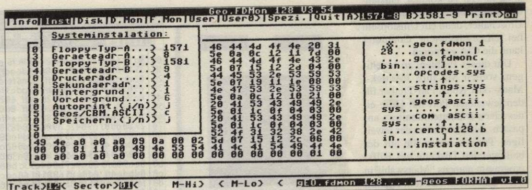
Die Oberfläche des GeoFDMon: Sehr übersichtlich durch 80 Zeichen
