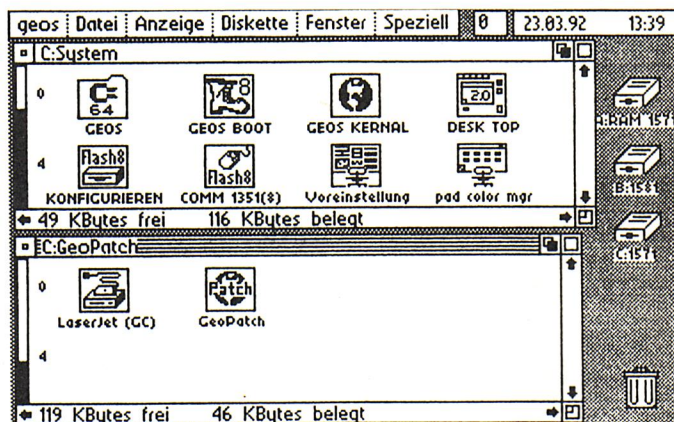
Wenn alles klappt, erzeugt das Geos-Patchprogramm für die BootDatei, "Konfigurieren" und den Maustreiber neue Icons
