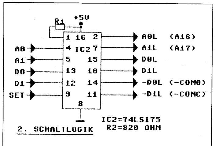
Bild 2. RAM-Schaltlogik
