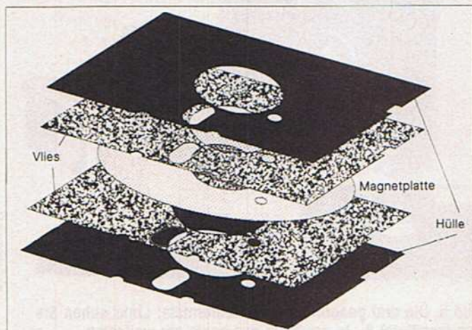
Bild 4. Schnitt durch eine handelsübliche 5¼-Zoll-Diskette
