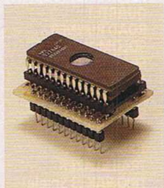
Bild 1. Ein Adaptersockel erlaubt das mühelose Auswechseln der Bausteine im Computer
