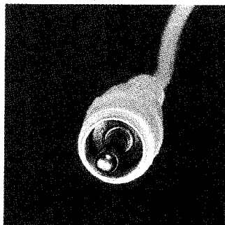
Bild 1. Cinch-Stecker, wie sie viele Monitore (z. B. der 1702) verwenden
