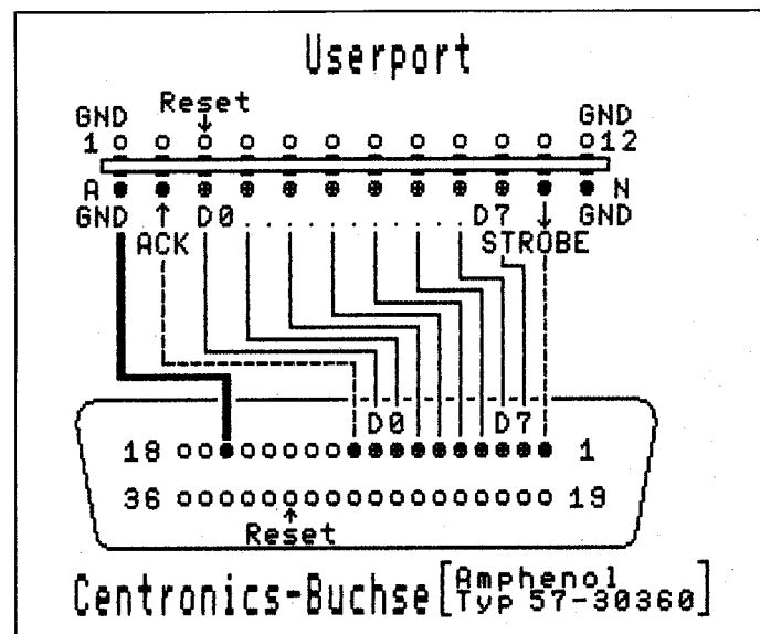
Bild 1. Verbindungskabel User-Port/Centronics-Schnittstelle
