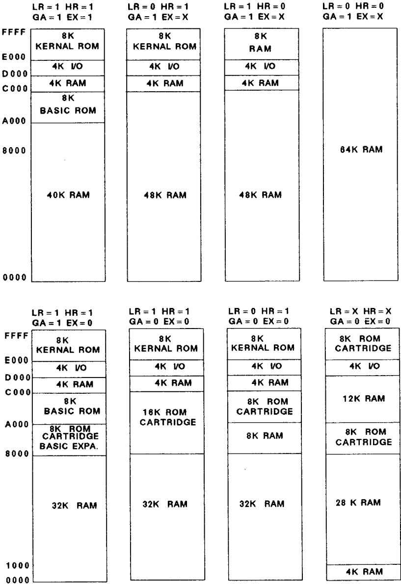
LR = LORAM HR= HIRAM GA=GAME EX=EXROM Abb. 6.5.1.2: Speicheraufteilung
